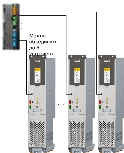
Рис. 3-2 Параллельное соединение базовых выпрямительных блоков
