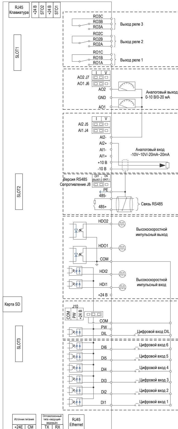
Рис. 3-3 Проводка контура блока управления
