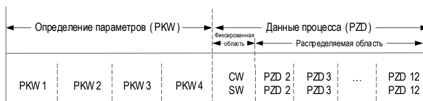
Рис. 8-1 Структура сообщения
