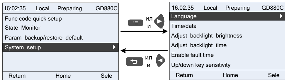
Рис. 4-17 Системные настройки
