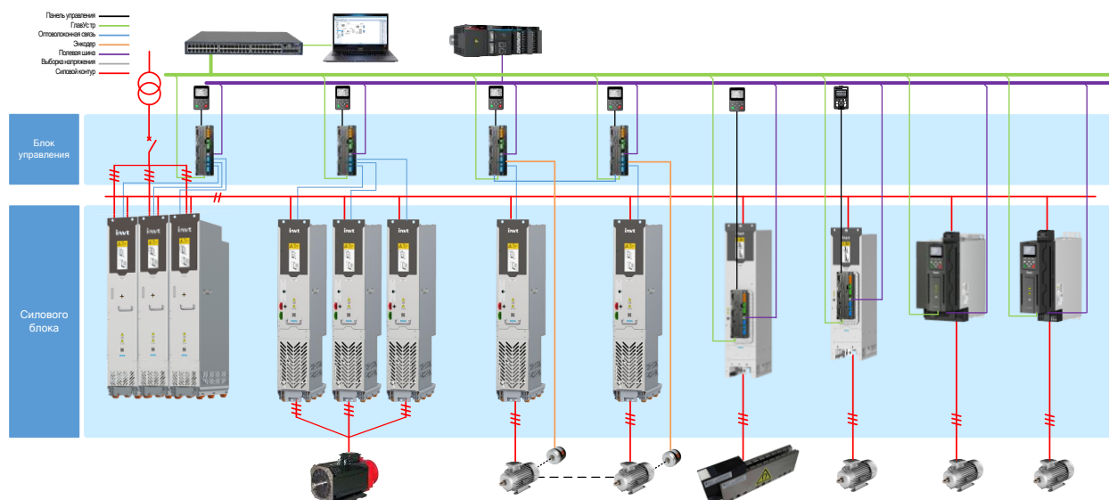
Рис. 3-1 Типовая топология мультипривода GD880
