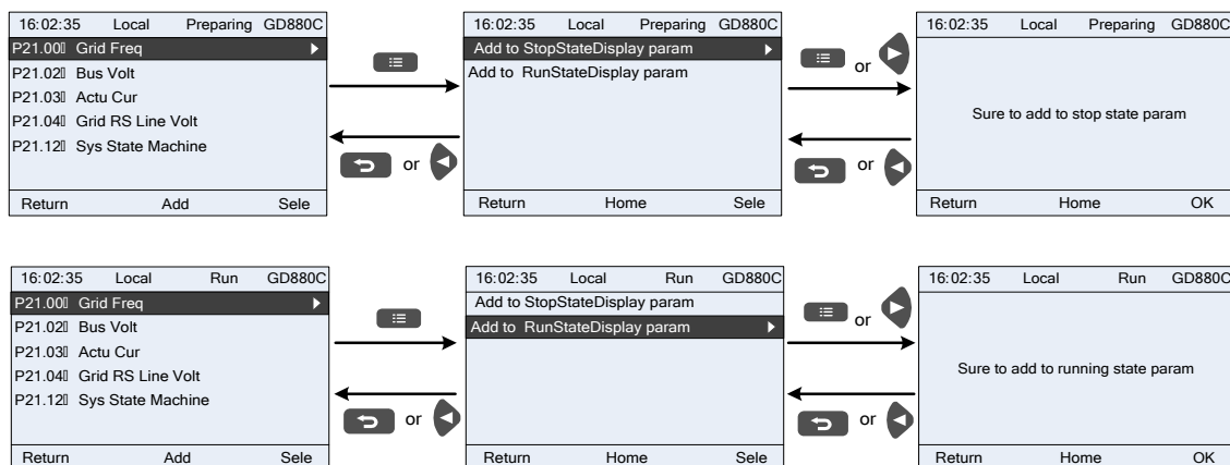
Рис. 4-12 Добавление параметров
